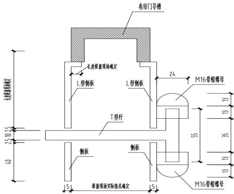
图1 施工图
