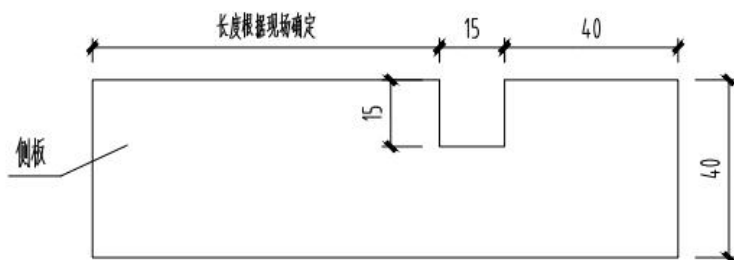
图3 施工图
