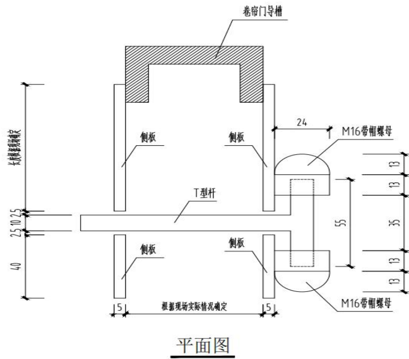
图1 施工图
